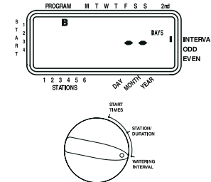
Ilustración 8: Pantalla LCD con intervalo de riego
