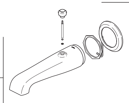
RP78581▲ Tub Spout/Pull-Up Diverter Tubo de salida para bañera/ botón desviador de alzar Bec/avec dérivation à tirette
