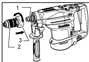
1. Eje 2. Mandril de cambio rápido 3. Cubierta de cambio
