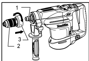
1. Axe 2. Mandrin à adaptateur rapide 3. Couvercle adaptateur
