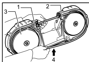
1. Support supérieur 2. Support inférieur 3. Meule 4. Appuyer
