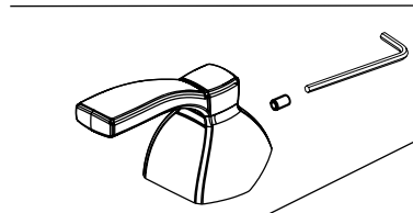
RP101044▲ Handle Kit Conjunto de manija Montage de la manette
