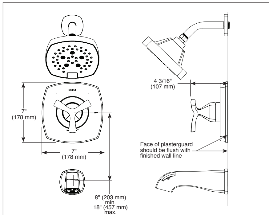
RP93376▲ (Pull-Up Diverter)
