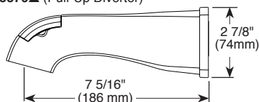
RP93376▲ (Pull-Up Diverter)
