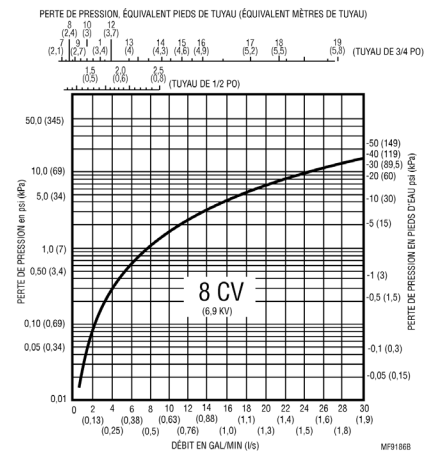
Fig. 2c. Caractéristiques de débit de la vanne de 8 Cv (6,9 kW).
