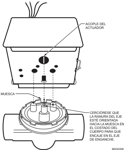
Fig. 2. Instalación del actuador nuevo.
