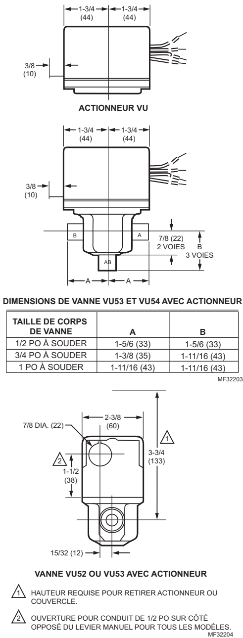
Fig. 1. Dimensions de montage en po (mm).
