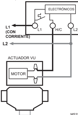
Fig. 4. Cableado típico para el actuador de la serie VU40.
