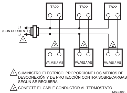
Fig. 5. Conexiones del actuador serie VU80 y del termostato serie T822.
