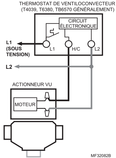
Fig. 4. Câblage typique de l'actionneur série VU40.
