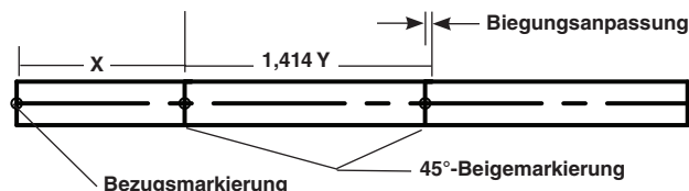
A – Ungebogenes Rohr mit Markierungen
