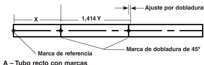
A – Tubo recto con marcas
