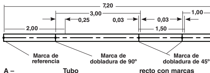
A – Tubo recto con marcas
