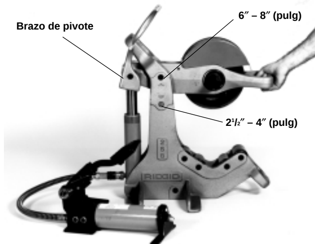
Figura 10 – Regulación del brazo de pivote
