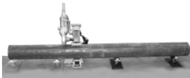
Figura 7A – Tubo largo
