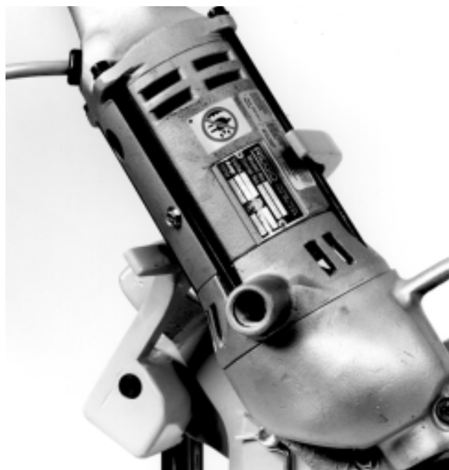
Figura 5 – Coloque el Accionamiento motorizado dentro del brazo de reacción
